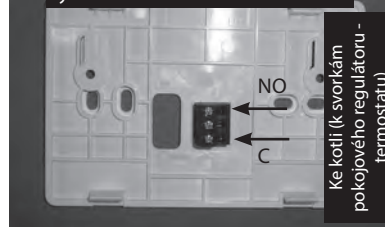
Využití kontaktu v Exeotermostatu
